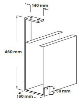
STAFFA A SOFFITTO CON TRAVE
