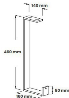
STAFFA A SOFFITTO
