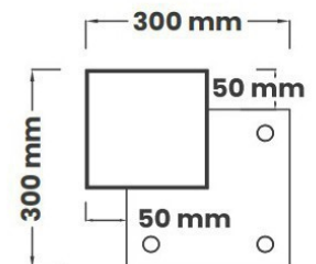
PIASTRA DI BASE TIPO D: predisposizione per montaggio Clear
