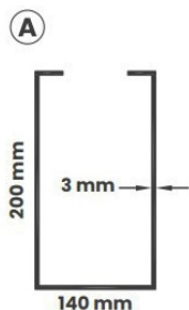
Trave perimetrale lato alto
