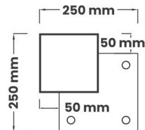
PIASTRA DI BASE TIPO D: predisposizione per montaggio Clear
