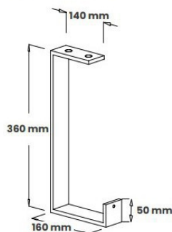
STAFFA A SOFFITTO
