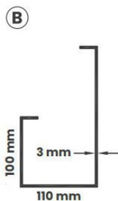
B Trave perimetrale lato basso
