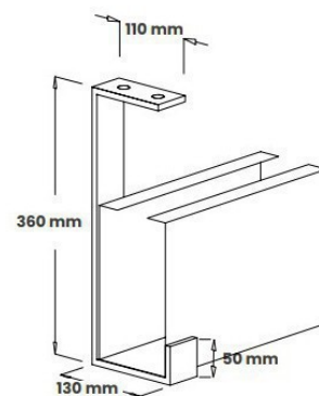
STAFFA A SOFFITTO CON TRAVE
