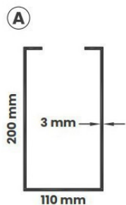
A Trave perimetrale lato alto
