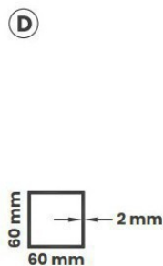
D Profilo rompitratte
