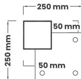
PIASTRA DI BASE TIPO D: predisposizione per montaggio Clear
