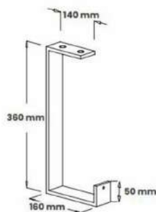
STAFFA A SOFFITTO
