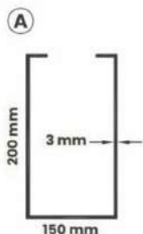
Trave perimetrale lato alto
