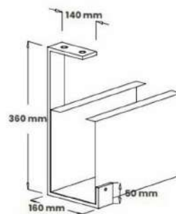
STAFFA A SOFFITTO CON TRAVE
