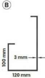
Trave perimetrale lato basso
