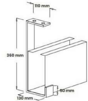
STAFFA A SOFFITTO CON TRAVE
