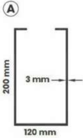
Trave perimetrale lato alto
