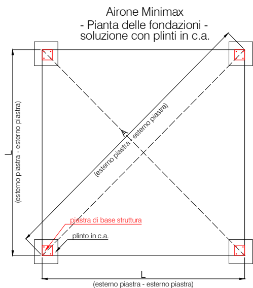
Dimensioni e peso dei plinti/zavorre necessarie per ogni piantone
